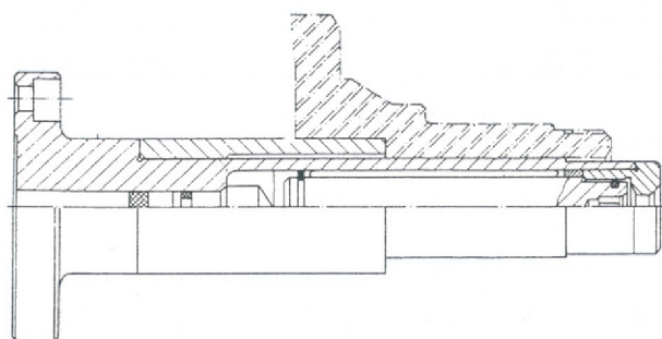
Mandrini ad espansione con rullini per lavorazioni di precisione e collaudi
