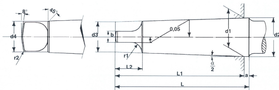
Attacco cono morse - forma B - DIN 228
