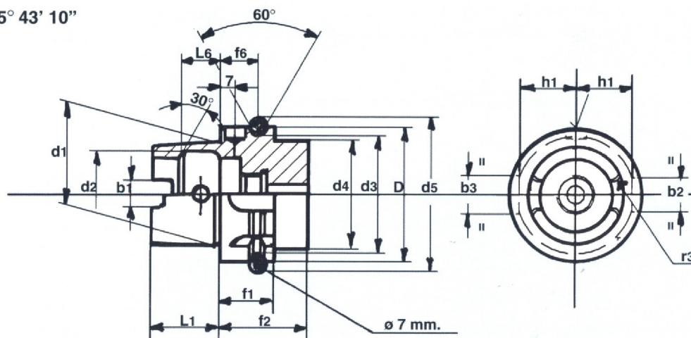
Dimensioni principali
