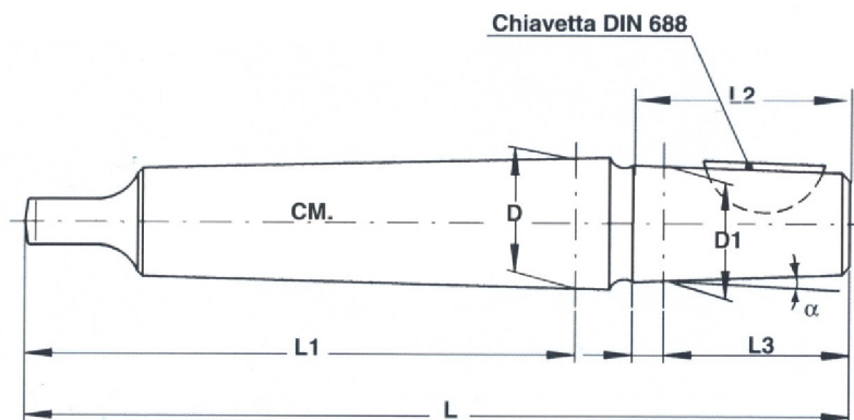
Attacco conico - DIN 238 con chiavetta e codulo CM. Tipo B
